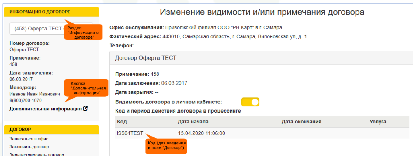
Рис. 4. Окно интерфейса настроек процессинга топливных транзакций. ООО "РН-Карт".
